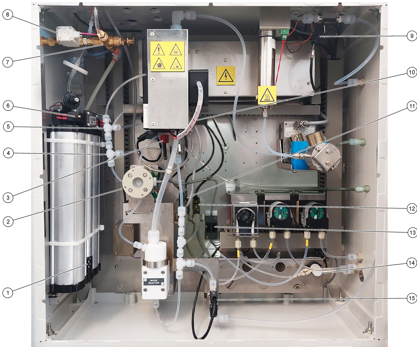
Figur 3 Analysekabinettets ventiler
